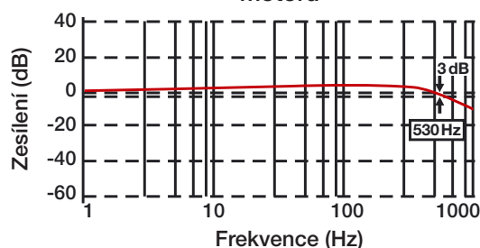
Bodeův diagram pro 0,75kW setrvačnost zátěže = setrvačnost motoru
