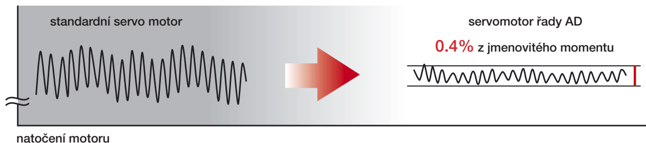
Příklad standardního motoru 0.75 kW Torque
