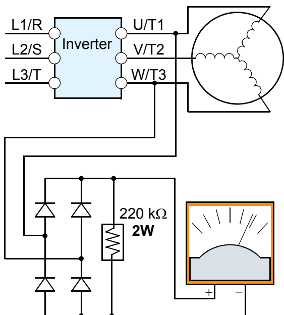
Měření napětí se zátěží
