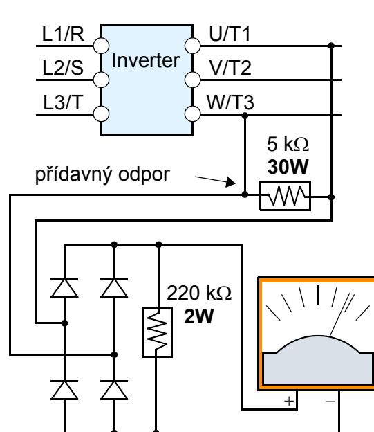
Měření napětí bez zátěže
